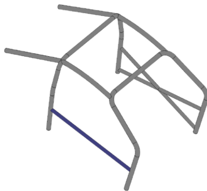
En vue de côté, l'inclinaison de l'entretoise est autorisée.
