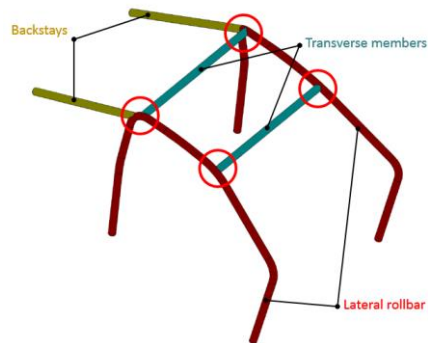
Dessin/Drawing SC-3
