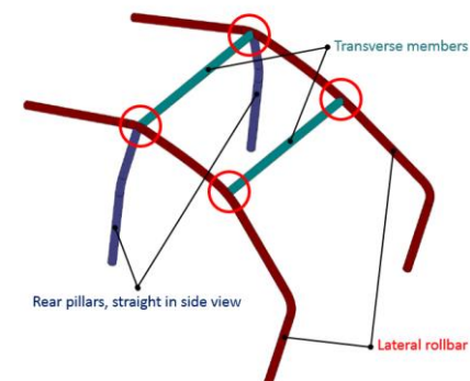
Dessin/Drawing SC-3
