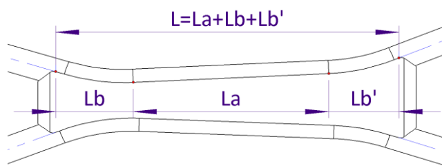
Bords avant et arrière rectilignes Straight front and rear edges
