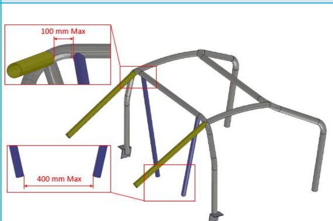
Dessin/Drawing SC-6b
