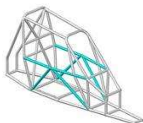
Dessin / Drawing 279B-10
