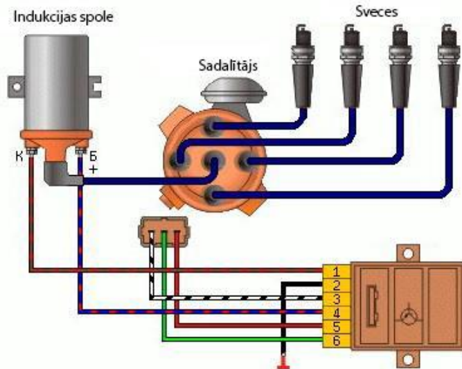
3.att. Elektroniskās aizdedzes shēma.
